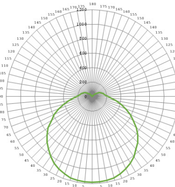
LLS360-35-40-LV-XX
