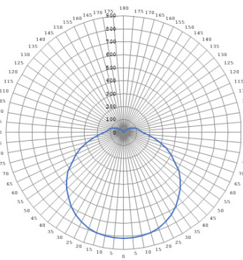
LLS360-25-40-LV-XX
