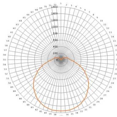
LLS360-47-40-LV-XX
